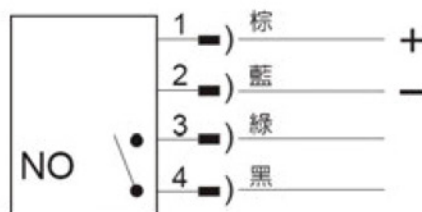
繼電器輸出型(NO)
